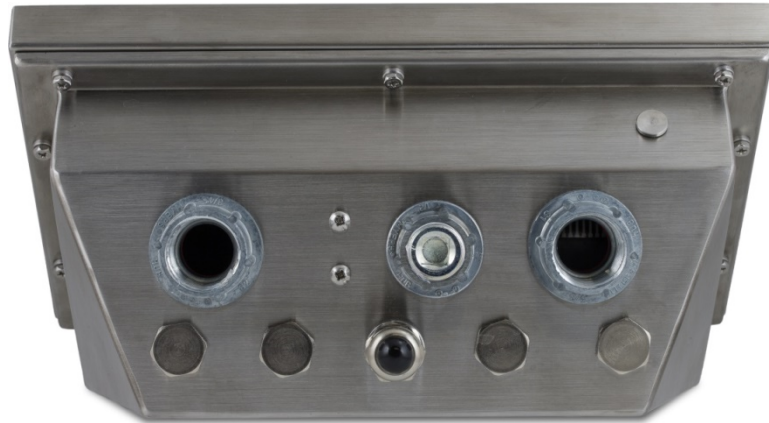
Abbildung 2-1: Kabeleinführungen
