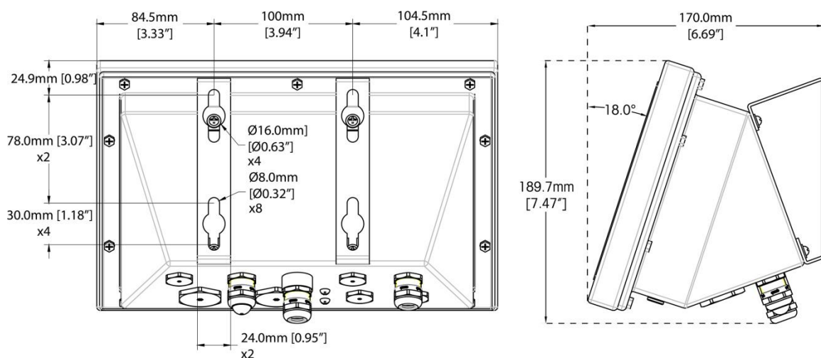
图 1-7: IND570xx 防尘式结构尺寸，配备 VESA 标准固定安装支架
