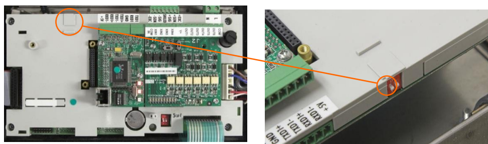
图 5-29：开关 SW2-1 的位置
