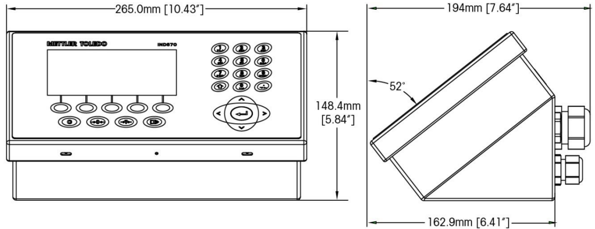
图 1-5: 防尘式结构尺寸
