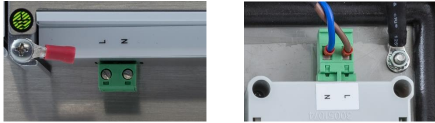
图 5-13: 交流电测试点—面板（左）和防尘（右）
